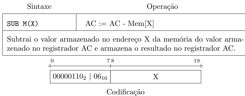
Figura 5.9: Instrução SUB M(X)
