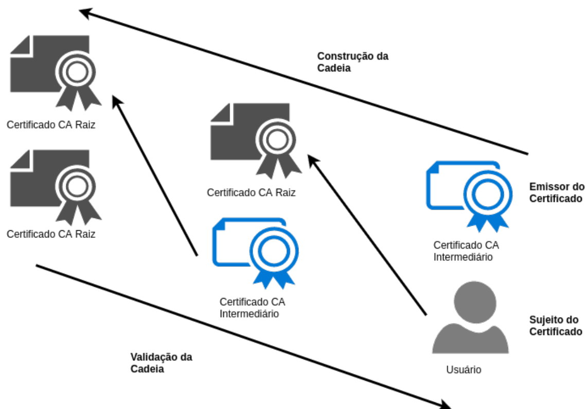
Figura 2. Modelo de Relações de Confiança
