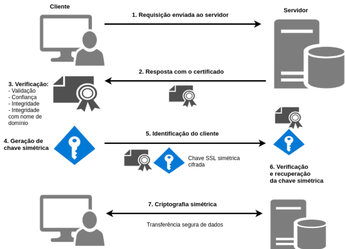
Figura 1. Funcionamento do SSL
